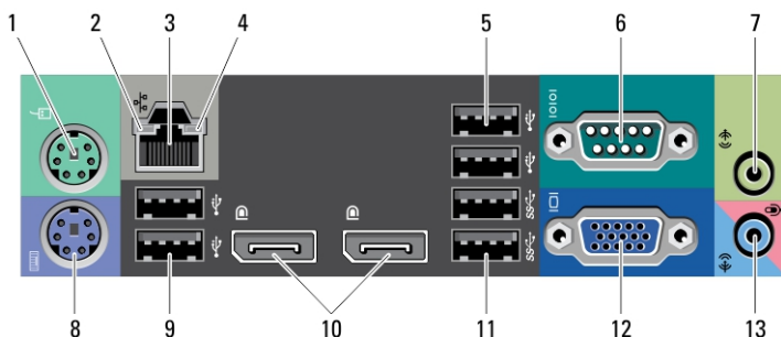
圖 2. 背面板視圖
