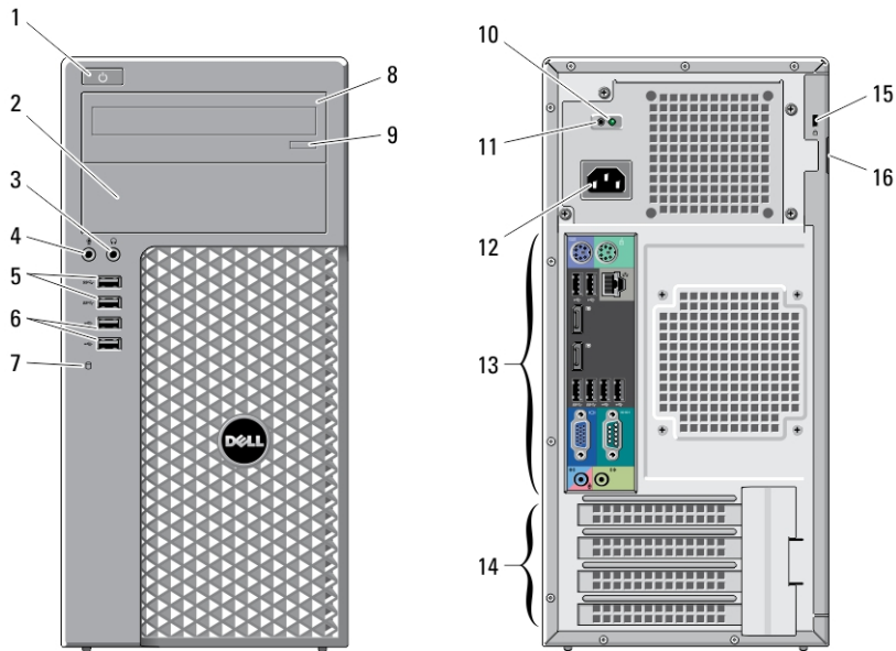
圖 1. 前視圖和後視圖
